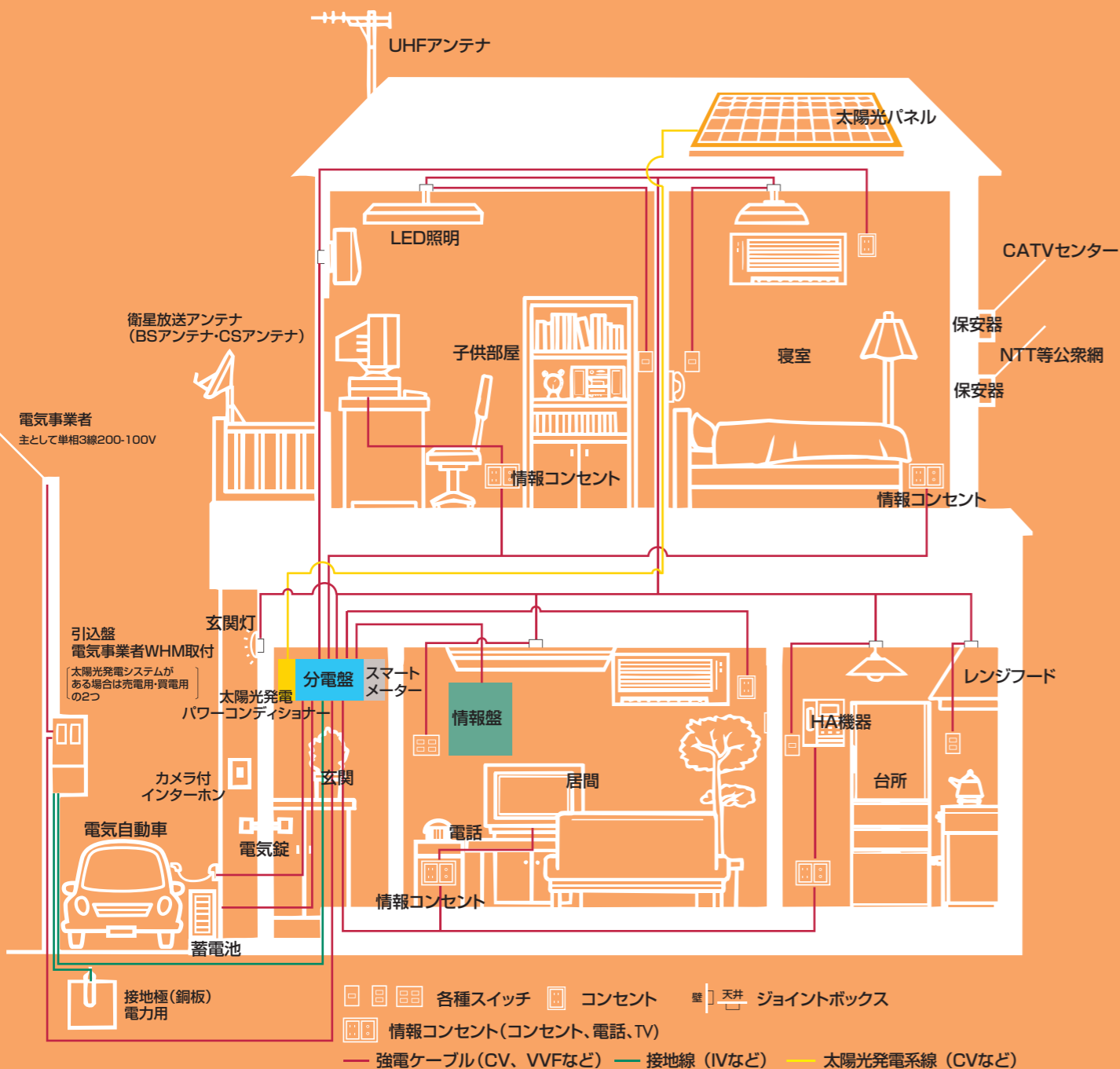
【住宅電力配線の仕組み】
