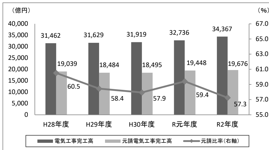
電気工事完工高と元請比率の推移
